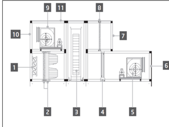
Рисунок 1: Образец схемы АНУ №1
