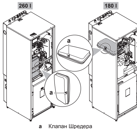
а Клапан Шредера
