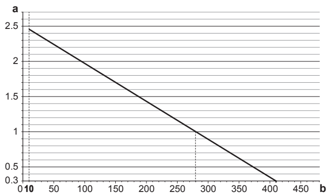
a Предварительное давление (бар) b Максимальный объем воды (л)
