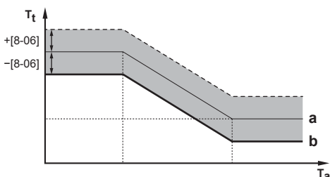
а Кривая зависимости от погоды
