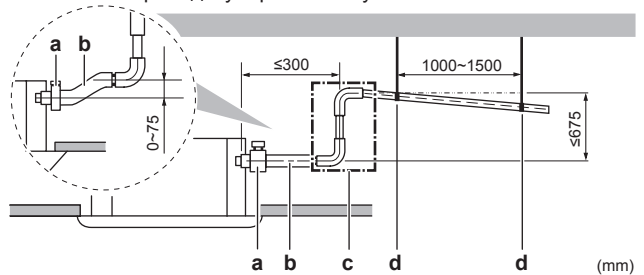
a Металлический зажим (входит в комплект принадлежностей) b Сливной шланг (входит в комплект принадлежностей) c Сливной трубопровод, направленный вверх (виниловая трубка с внутренним диаметром 25 мм и наружным диаметром 32 мм) (приобретается на месте). d Подвесные планки (приобретаются на месте)
