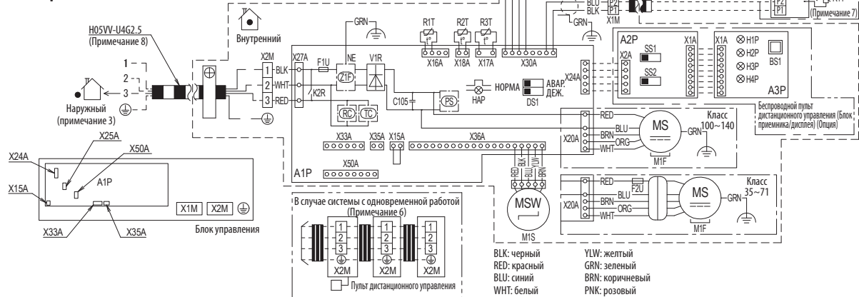
FHA-A(9) Электрическая схема
