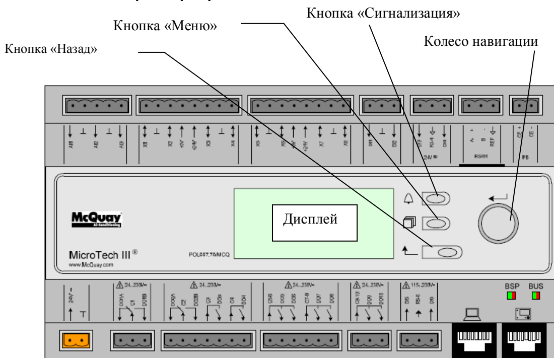
Рис. 6. Контроллер агрегата
